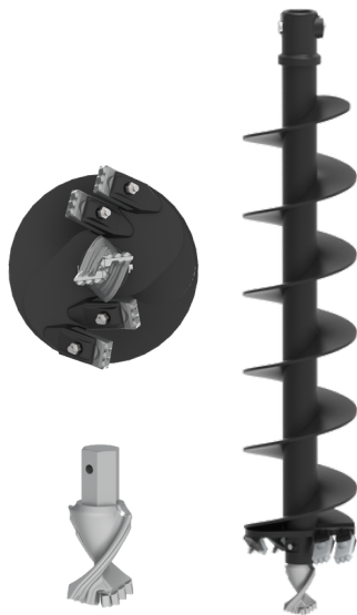
W2 D200 / D300 / D500 L1200 / L1500 / L1750 Soft Rock
